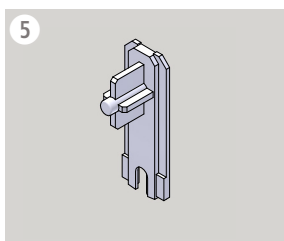
900 4417 28-3813-K***-W0 Blokada zatyczki lewej DC38 DC38 end cap left inside parts Замок крышка правой DC38 20 szt. 0,1 kg
