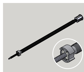
28-3826-K4417-W2 Sprężyna z kontrolerem DC38 S2000 szara Spring + controller DC38 S2000 grey Пружина с контроллером DC38 S2000 серая 2 szt. 0,65 kg
