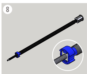
28-3826-K0517-W3 Sprężyna z kontrolerem DC38 S3000 niebieska Spring + controller DC38 S3000 blue Пружина с контроллером DC38 S3000 синяя 2 szt. 0,7 kg
