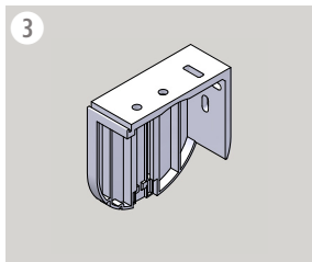
900 4417 28-3811-K***-W0 Zatyczka lewa DC38 DC38 end cap left Крышка лева DC38 20 szt. 0,65 kg
